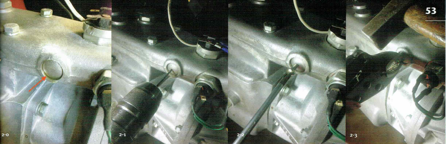
Lekkage bij de vriesdop
