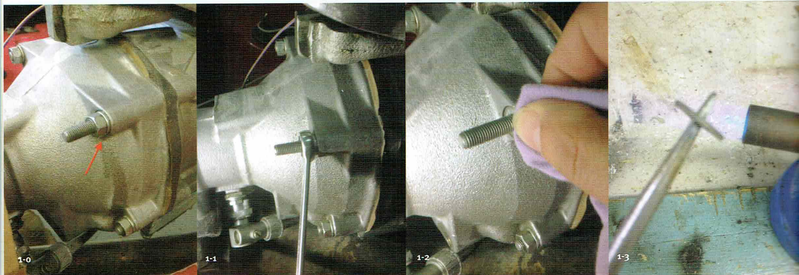
Lekkage langs de tapeinden J-Type overdrive
